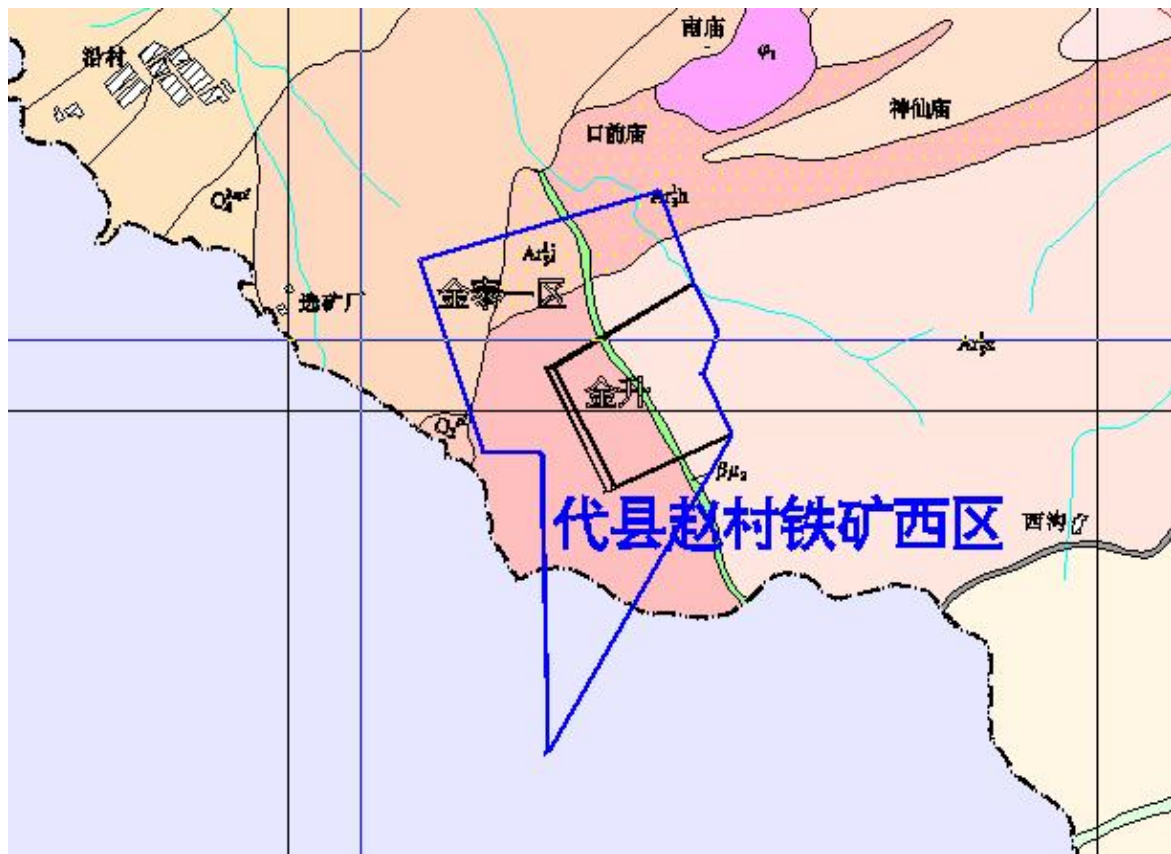
图 4-1 代县赵村铁矿西区
